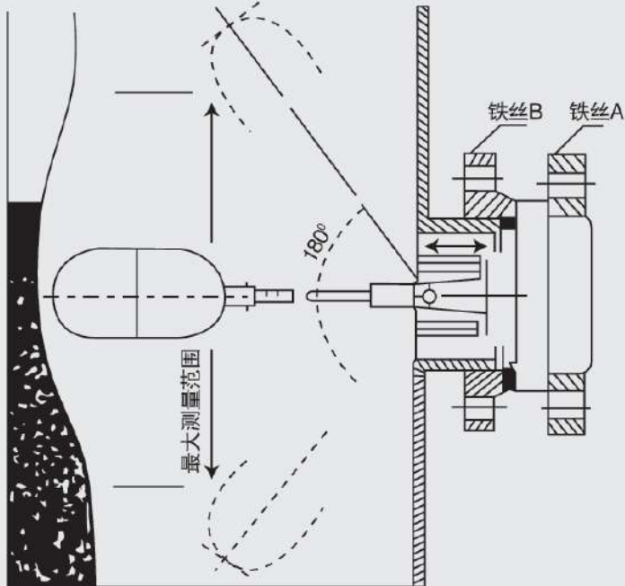
图三 UQZ-2型安装形式示意图
