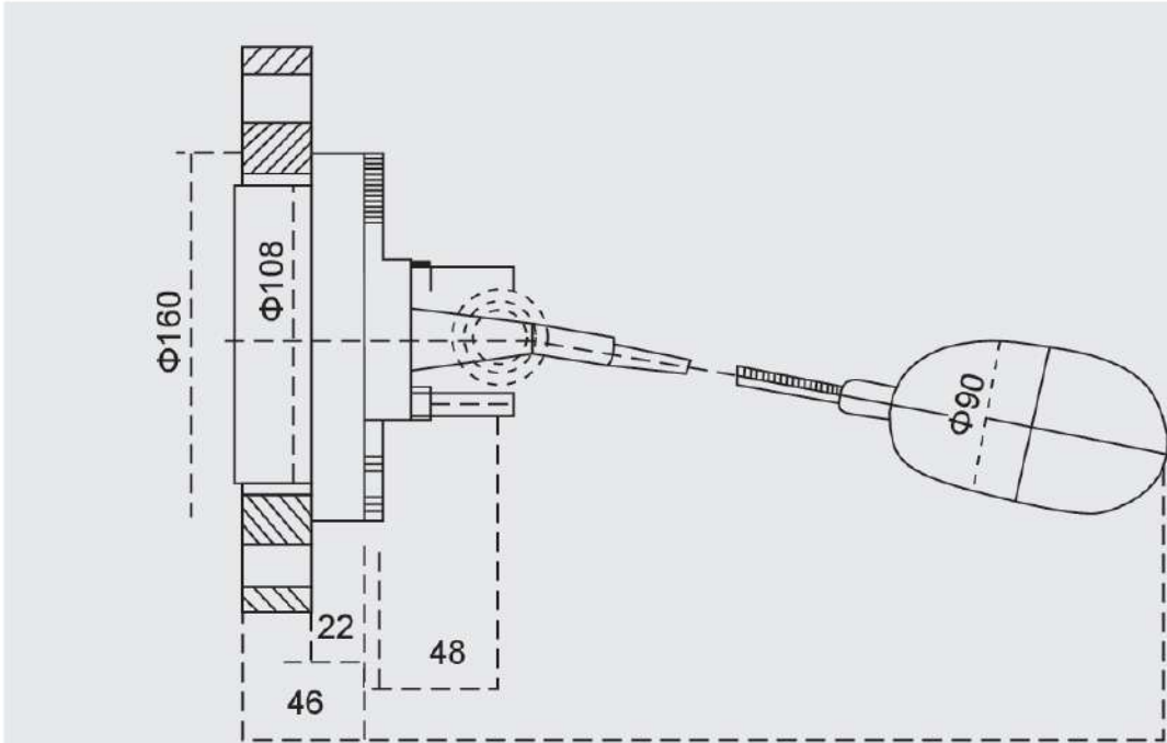
图二 UQZ-2型外形尺寸
