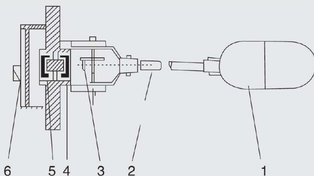
图一 UQZ-2 型结构原理图
