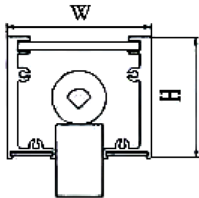
防霜型
